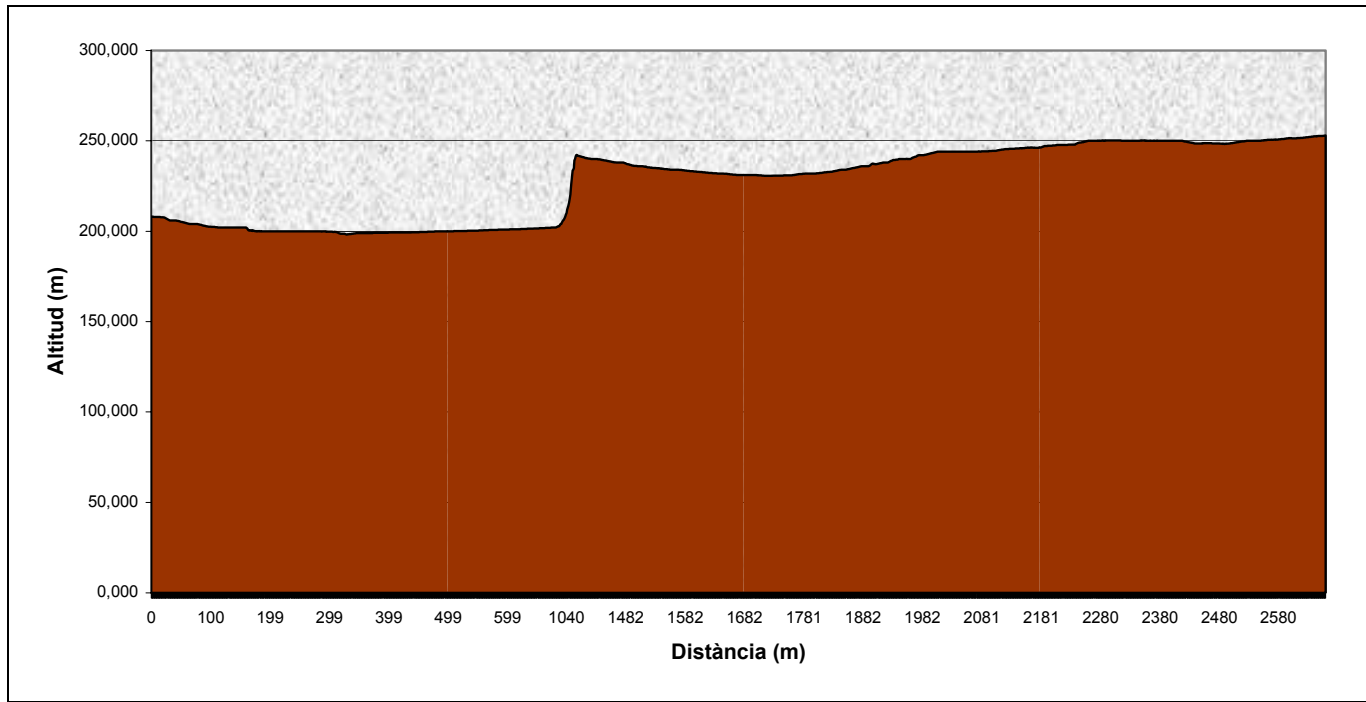
Perfil longitudinal del camí de les Cabanyes i Camí de la Pelegrina
