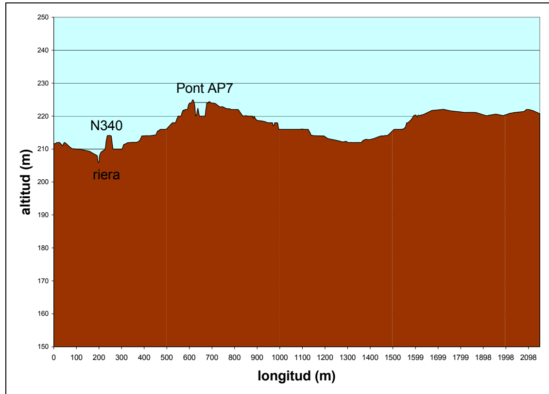
Perfil longitudinal del Camí de Meliό
