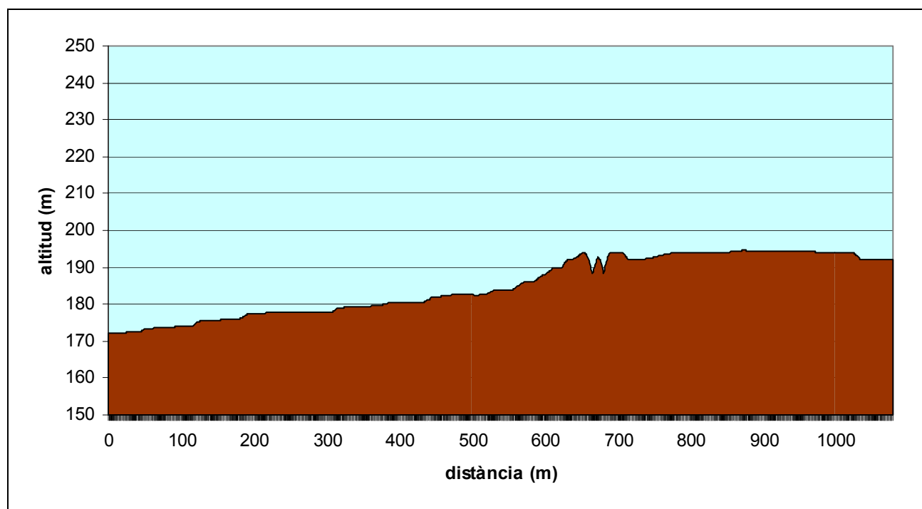
Perfil longitudinal del Camí de la Casa Nova
