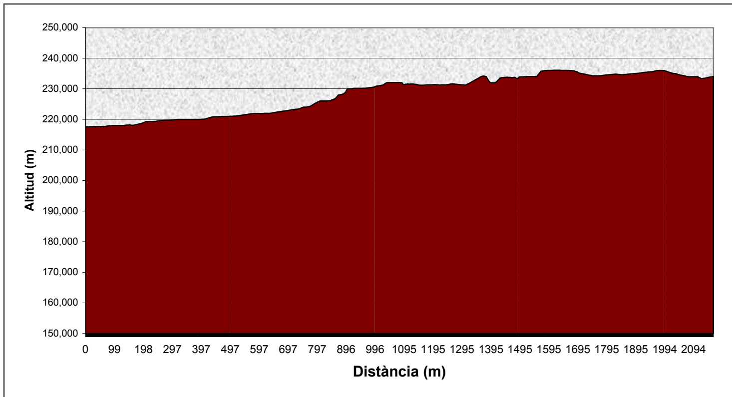
Perfil longitudinal del Camí de l'Hort del Tona (a partir del pas del LAV, inclòs tram d'Olèrdola).
