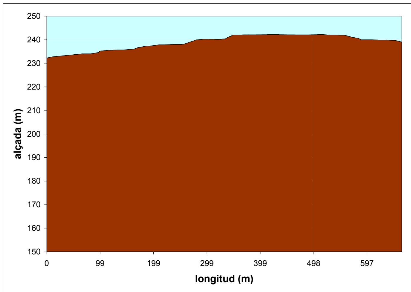
Perfil longitudinal del Camí lateral nord de l'AP-7 de Porroig a La Granada
