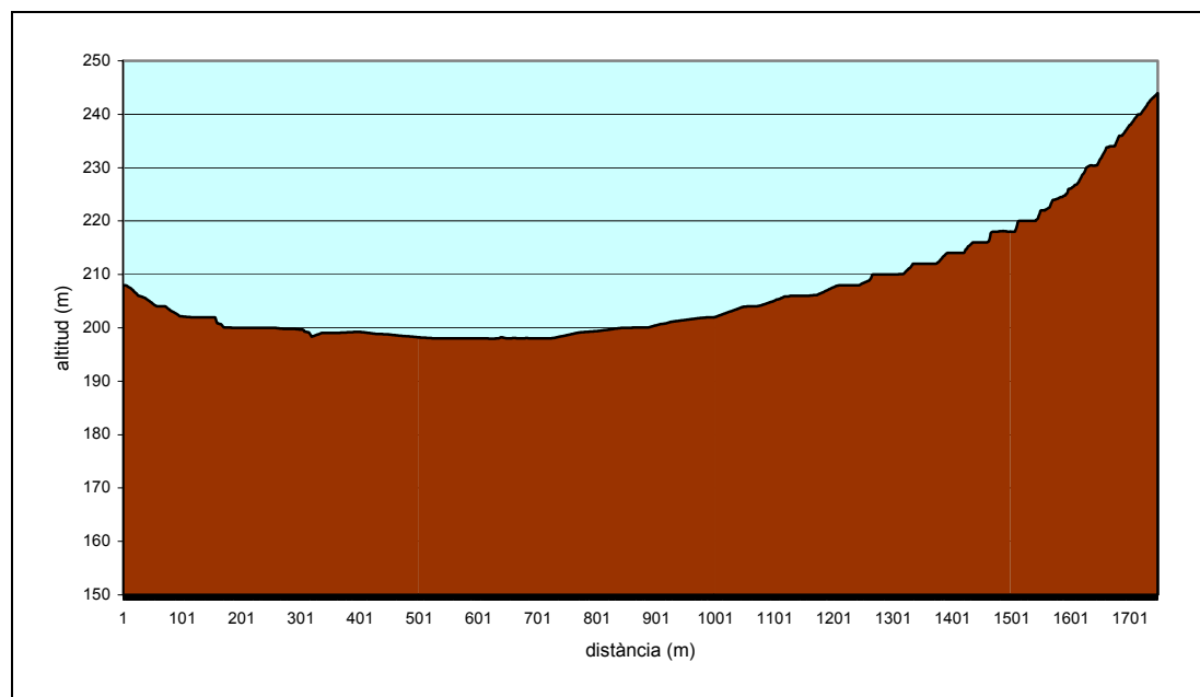
Perfil longitudinal del camí de Pacs
