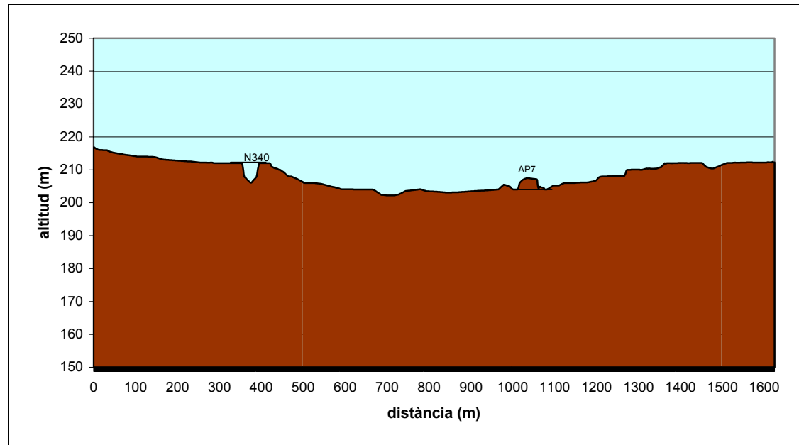
Perfil longitudinal del Camí de Mas Rabassa
