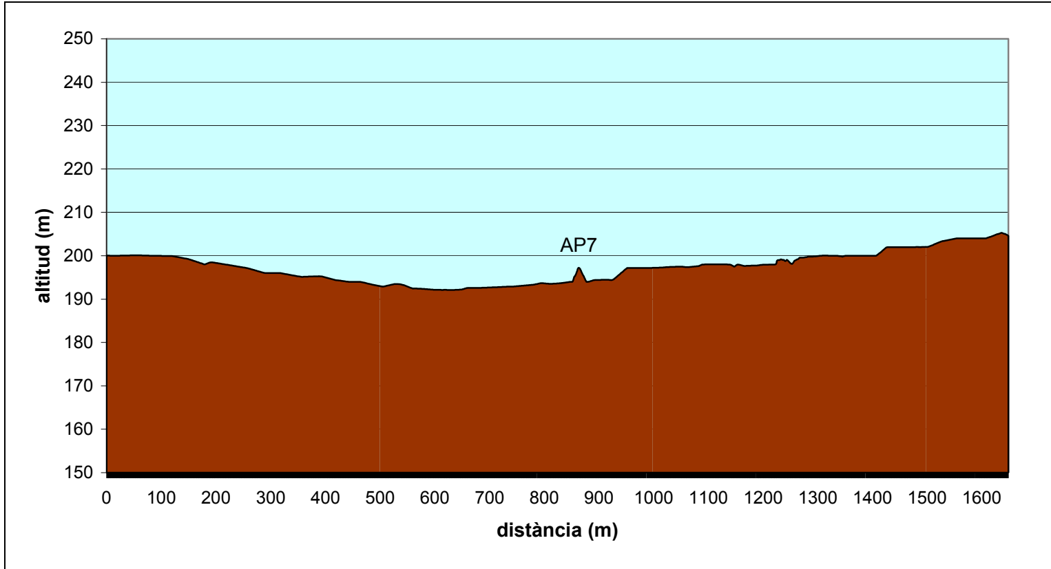
Perfil longitudinal del Camí de Moja a Sant Digna
