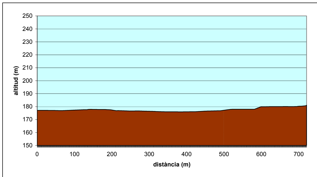
Perfil longitudinal del camí de Cal Sebeta
