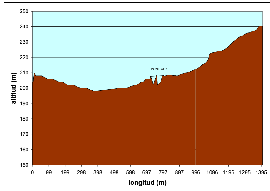
Perfil longitudinal del Camí de la Serreta o del Sant Sepulcre
