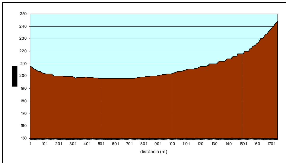
Perfil longitudinal del camí de la Sort
