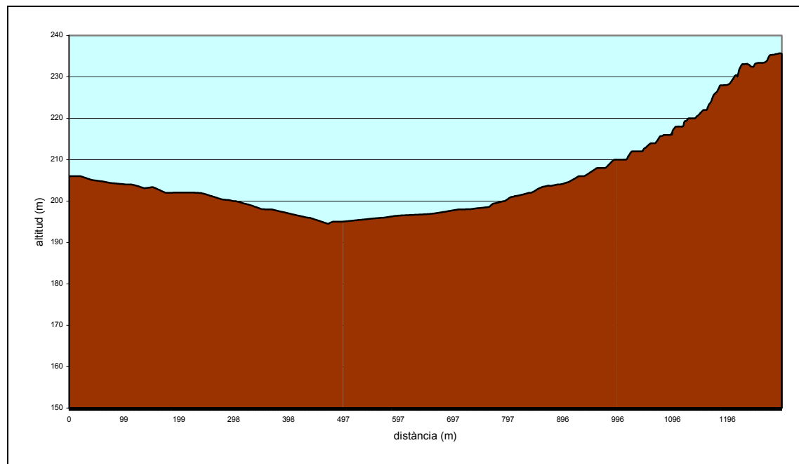
Perfil longitudinal del camí de Sant Pau 2
